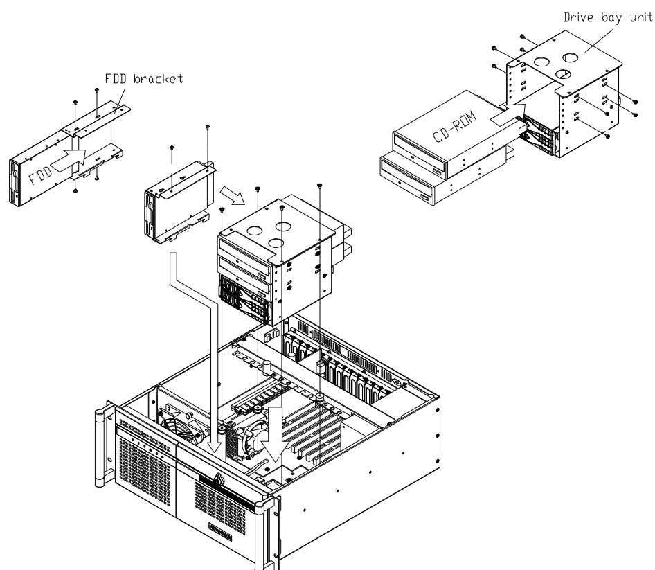
Figure 2.7 Installing Disk Drives/ 安装磁盘驱动器 / 安裝磁碟機
