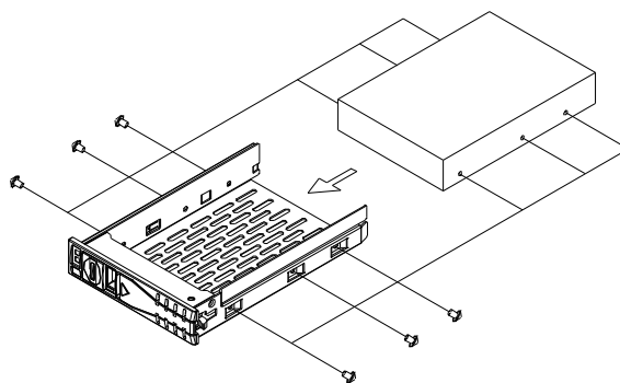
Figure 2.8 Installing a SATA HDD/ 安装 SATA 硬盘 / 安裝 SATA 硬碟
