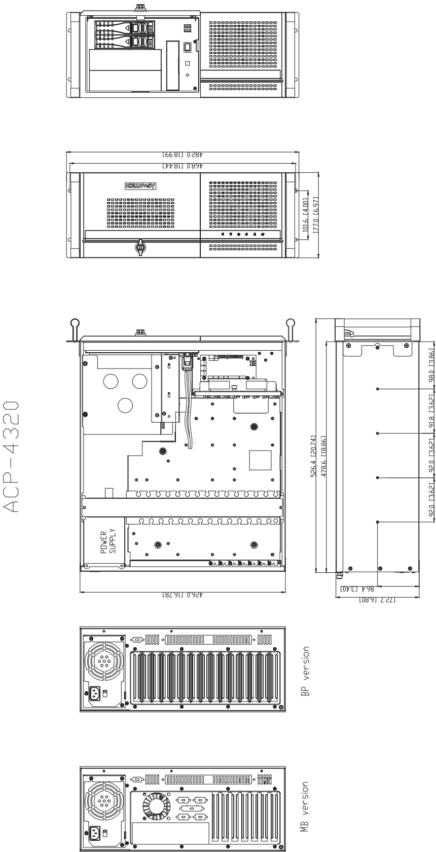
Figure 1.1 Dimensions Diagram/ 产品尺寸 / 產品尺寸
