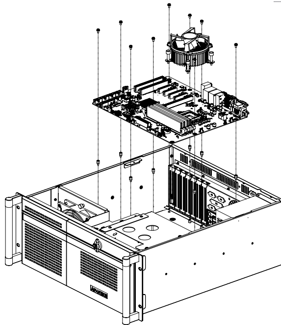
Figure 2.4 Installing a Motherboard/ 安装主板 / 安装主机板
