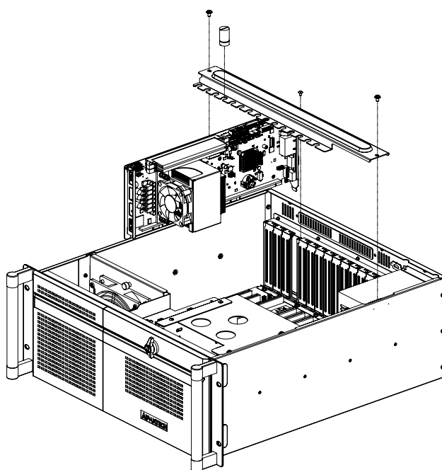
Figure 2.5 Installing a CPU card/ 安装 CPU 卡 / 安裝 CPU 卡
