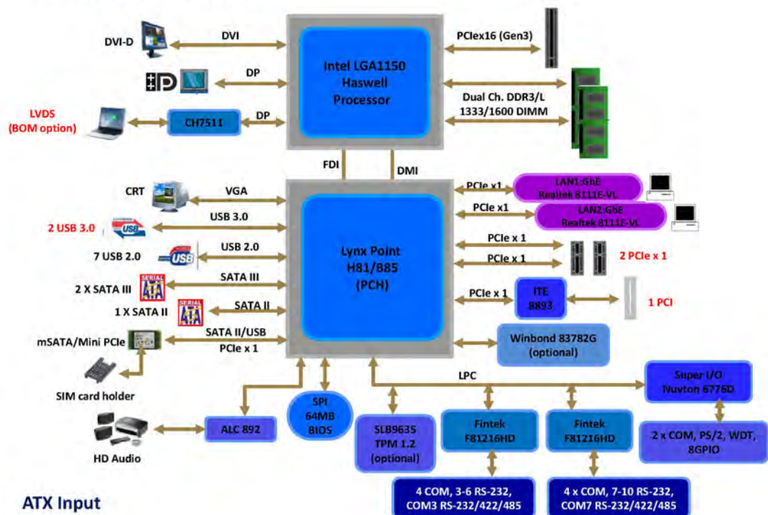
AIMB-503G2-00A1E (H81)
